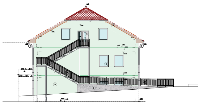
POHLED BOČNÍ (SV)
