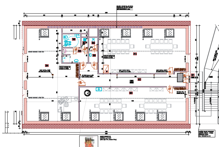
PŮDORYS PODKROVÍ
